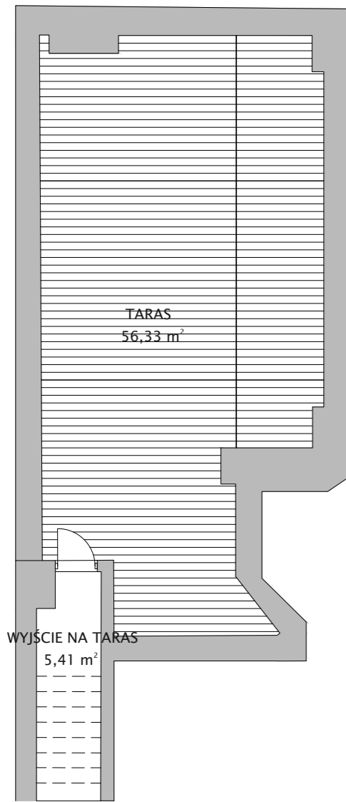
Rzut tarasu
